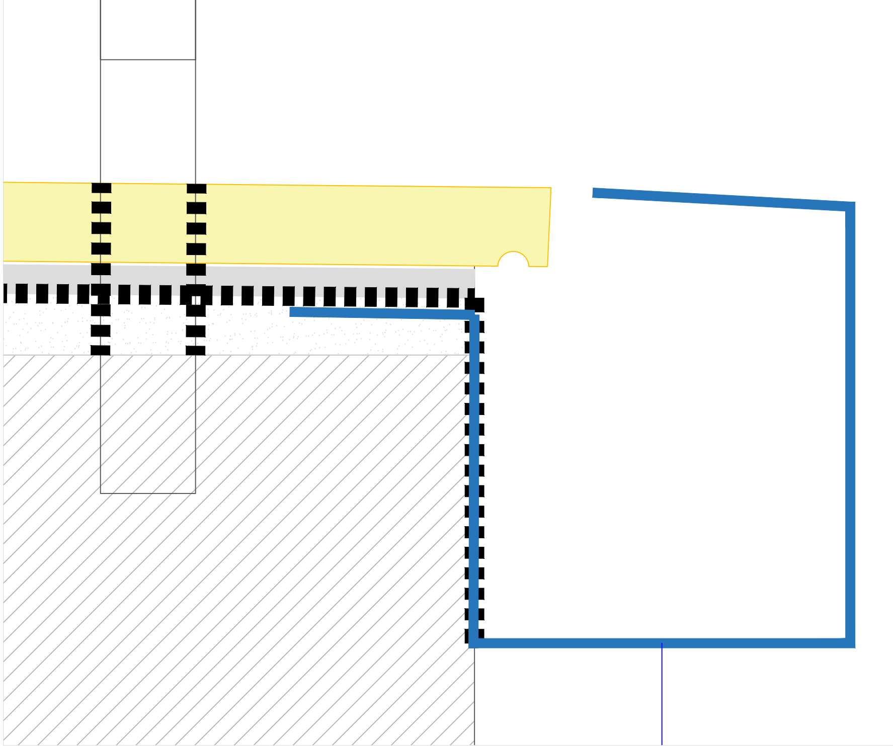
DETALLE CANAL Y ANCLAJE BARANDILLA ESCALA: 1/2
