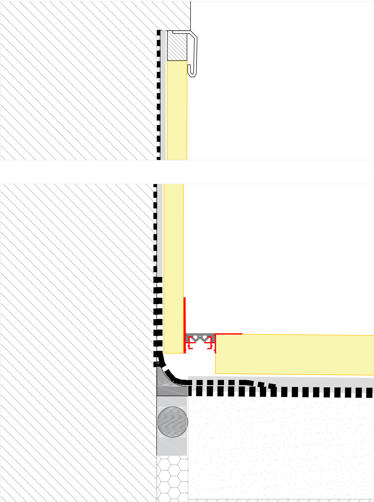
DETALLE JUNTA ESTRUCTURAL ESCALA: 1/2
